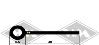
14118 Dachauflageprofil ZT EUR 4,90/m*
