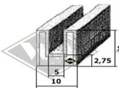
Samtschienen S23 5/10 mm EUR 5,80/m* S25 5/12 mm EUR 6,05/m* S26 5/13 mm EUR 6,55/m*
