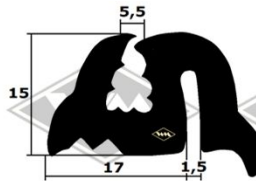
2069 Frontscheidenprofil feststehende Scheibe Heckscheidenprofil EUR 4,40/m*
