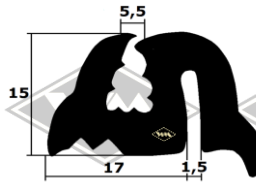
2069 Frontscheibenprofil feststehende Scheibe Heckscheibenprofil EUR 4,25/m*
