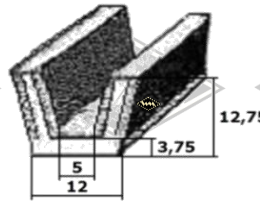
Samtschienen (Glas/Rücken) S25 5/12 mm EUR 5,50/m* S26 5/13 mm EUR 5,70/m* S30 6/12 mm EUR 5,95/m* S32 6/14,5 mm EUR 6,25/m*
