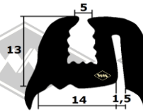
2375 Frontscheibenprofil feststehende Scheibe Heckscheibenprofil EUR 4,20/m*
