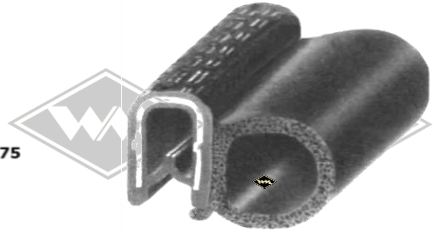
5001 Türabdichtung Klemmbereich 1,5-3,5 mm Wulst ca. 14 mm EUR 4,10/m*
