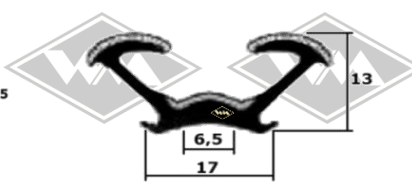
S35 Samtschiene EUR 6,70/m*
