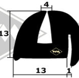
13100 Heckscheibenprofil alternativ EUR 5,70/m*
