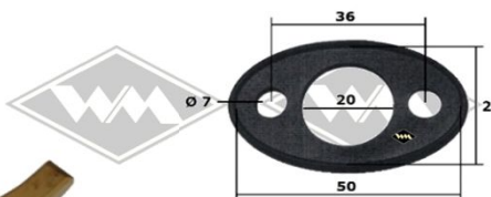
G81 Türgriffrosette klein Gummi
