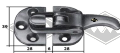
M73 Verdeckverschluß klein verchromt
