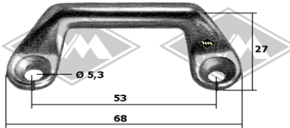
Türhalter-Krampe Gurtbreite 35 mm M53-1 schwarz lackiert M53-2 verchromt
