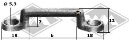
M51 Lakai-Krampe vernickelt Gurtbreite 25 mm
