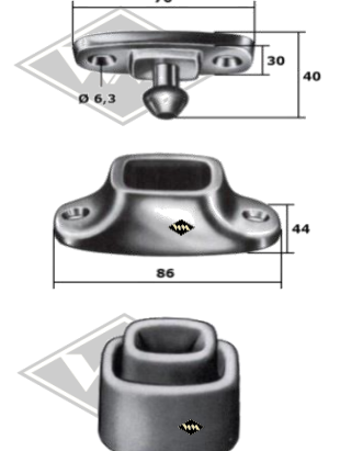
M76 Türfeststeller groß, 3-tlg. (Puffer 38x42 mm)
