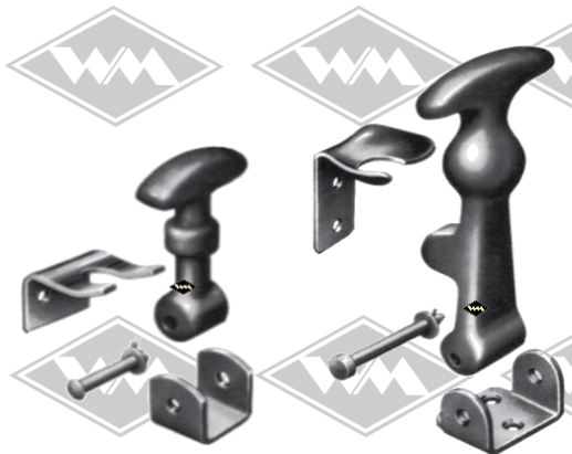
D94 Haubenhalter klein Gummiteil 64 mm
