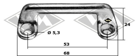
M55 Türhalter-Krampe verchromt Gurtbreite 40 mm
