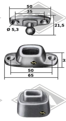
M77 Türfeststeller mittel, 3-tlg. (Puffer 30x26 mm)
