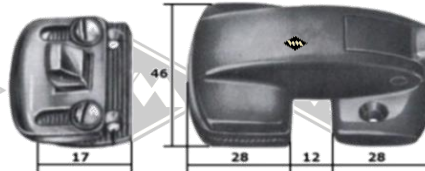
M74 Verdeckverschluß groß verchromt
