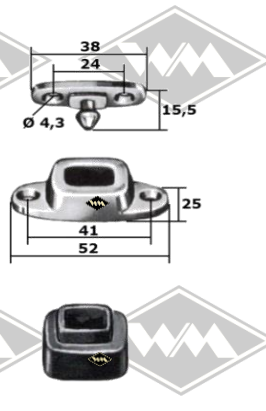
M75 Türfeststeller klein, 3-tlg. (Puffer 19x22 mm)
