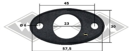
G82 Türgriffrossette groß Gummi
