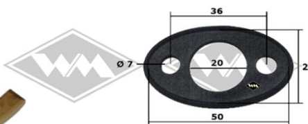
G81 Türgriffrossette klein Gummi
