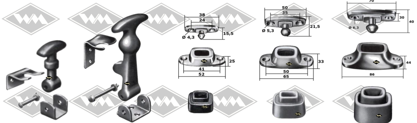
D94 Haubenhalter klein Gummitteil 64 mm
