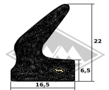
3321 Kofferklappen-/Hecktür- abdichtung Moosgummi EUR 4,00/m*
