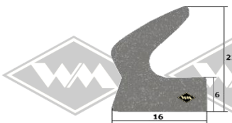
31676 Kofferklappen-/Hecktür- abdichtung Moosgummi alternativ grau EUR 4,00/m*
