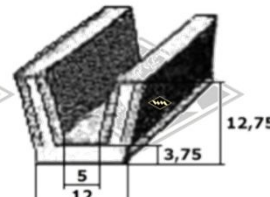
Führungsschiene S25 5/12 mm EUR 5,90/m* S26 5/13 mm EUR 6,35/m* S30 6/12 mm EUR 6,75/m*
