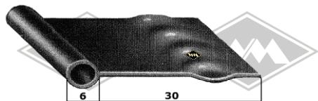
Kotflügelkeder P40 6/30 mm P45 9,5/28 mm
