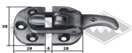
M73 Verdeckverschluß klein verchromt
