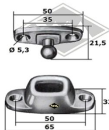
M55 Türhalter-Krampe verchromt Gurtbreite 40 mm
