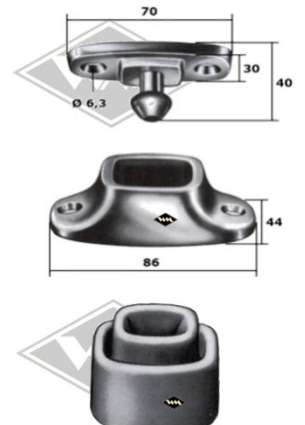
M76 Türfeststeller groß, 3-tlg. (Puffer 38x42 mm)
