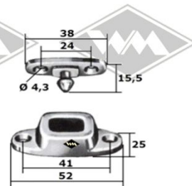
Türhalter-Krampe Gurtbreite 35 mm M53-1 schwarz lackiert M53-2 verchromt
