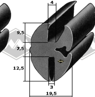
40109 Scheibenprofil Qek alternativ EUR 7,50/m*
