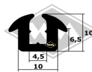
4040 Ausstellfenster innen u.a. Apolda, Friedel, Dübner Ei EUR 5,10/m*
