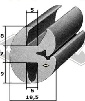
40114 Scheibenprofil Qek alternativ Füller: G55/P10 EUR 6,90/m*
