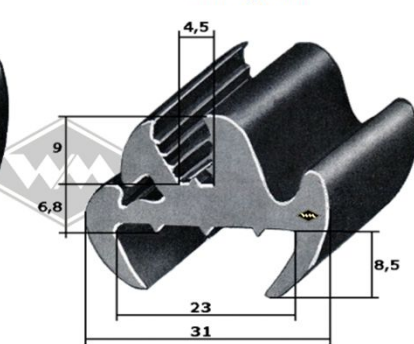
40152 Scheibenprofil u.a. QEK 325, Weferlinger, "Aller300", Mostard Yvonne HD306 Füller: G55/P10/P50 EUR 9,95/m*
