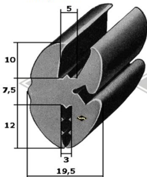
40113 Scheibenprofil Qek alternativ Füller: G55/P10 EUR 7,25/m*
