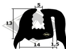
2375 Scheibenprofil u.a. Friedel EUR 5,60/m*
