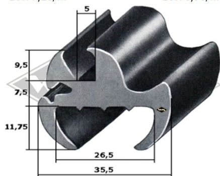
40153 Scheibenprofil u.a. QEK 325 Füller: G55/P10/P50 EUR 10,20/m*
