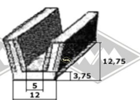
Samtschiene u.a. Dübener Ei S25 5/12 mm EUR 6,20/m* S30 6/12 mm EUR 7,20/m*
