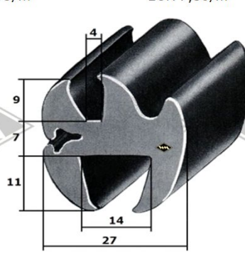
40151 Scheibenprofil Füller: G55/P10 EUR 11,85/m*
