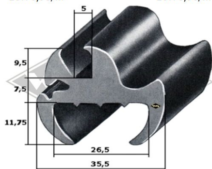
40153 Scheibenprofil u.a. QEK 325 Füller: G55/P10/P50 EUR 10,20/m*
