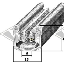
S119 Führungsschiene mit Metalleinlage EUR 7,90/m*
