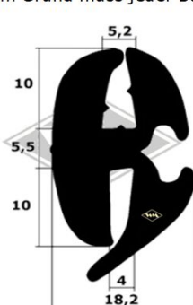
3557 Scheibenprofil Qek alternativ Füller: P10/P11 EUR 6,55/m*
