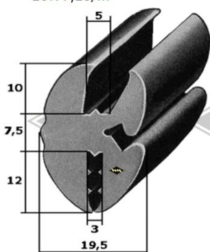
40113 Scheibenprofil Qek alternativ Füller: G55/P10 EUR 6,95/m*
