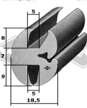
40114 Scheibenprofil Qek alternativ Füller: G55/P10 EUR 6,90/m*
