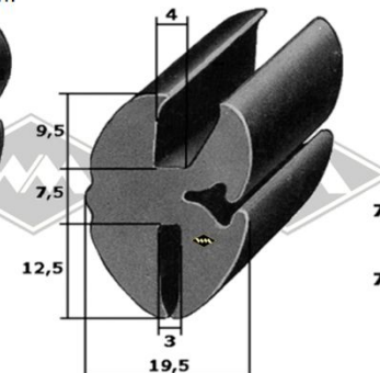
40109 Scheibenprofil Qek alternativ Füller: G55/P10 EUR 7,50/m*
