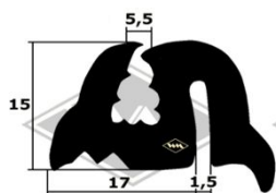
4084 Ausstellfenster u.a. Bastei, Dübener Ei, Friedel, Lausitz 310, Nagetusch, Weferlinger EUR 6,95/m*
