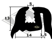
2375 Scheibenprofil u.a. Friedel EUR 5,30/m*
