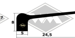
4009 Abdichtung Tür hinten B-Säule Fixlänge à 0,80 m EUR 8,50/Länge*
