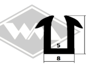
4004 Abdichtung Rundung Dreiecksfenster hinten Fixlänge à 0,56 m EUR 7,90/Länge*
