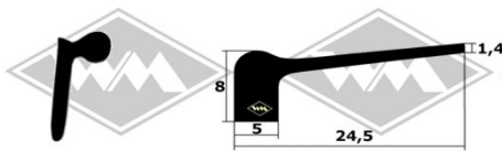
4005 Abstreifprofil innen EUR 2,95/m*
