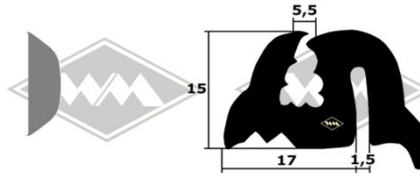
P6 Füllerprofil grau/schwarz für 1089/1089G EUR 1,60/m*
