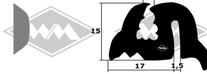
P6 Füllerprofil grau grau/schwarz für 1089/1089G EUR 1,60/m*
