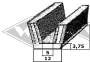
S25 Samtschiene 5 mm Glas / 12 mm Rücken EUR 5,50/m*
