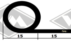
7486 Gummiprofil Schiene Türabdichtung unten, B-Säule EUR 3,80/m*
