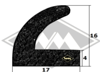
31029 Kofferklappen-/Hecktür- abdichtung Moosgummi alternativ EUR 3,80/m*
