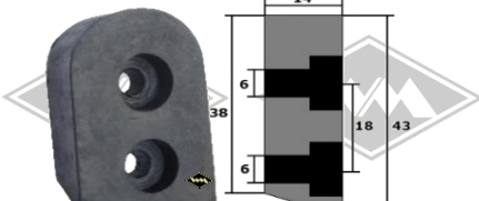
G35 Türfangpuffer abgerundet klein EUR 4,70/St*
