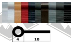
P8 PVC-Biese 4x10 mm transparent, weiß, terra- kotta, rot, dkl.blau, grün, braun, grau, anthrazit, schwarz EUR 1,50/m*
