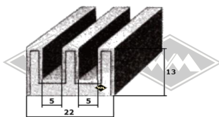
S37 Doppelte Samtschiene EUR 7,60/m*
