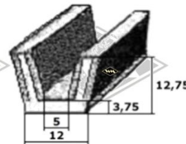
Führungsschiene S25 5/12 mr EUR 5,90/m* S26 5/13 mr EUR 6,35/m* S30 6/12 mr EUR 6,75/m*
