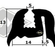
2375 Seitenscheibenprofil Limo+Kombi Heckscheibenprofil Kombi EUR 5,60/m*
