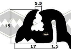
2069 (alternativ) Seitenscheibenprofil Limo+Kombi EUR 5,85/m*
