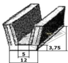
S25 Samtschiene 5 mm Glas / 12 mm Rücken EUR 8,40/m*
