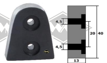
G22 Türfangpuffer keilförmig groß EUR 4,80/St*
