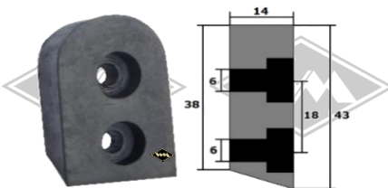
G35 Türfangpuffer abgerundet klein EUR 4,70/St*
