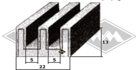
S37 Doppelte Samtschiene EUR 9,60/m*
