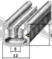
S125 Samtschienen mit Metalleinlage EUR 5,65/m*
