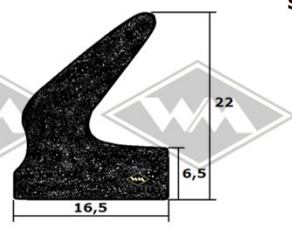
3321 Türabdichtung EUR 4,00/m*
