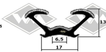
S35 Samschiene EUR 6,70/m*
