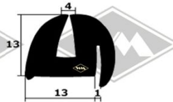
13100 Heckscheibenprofil EUR 5,70/m*
