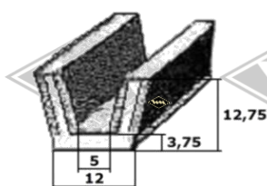
Samtschienen (Glas/Rücken) S25 5/12 mm EUR 6,20/m* S26 5/13 mm EUR 6,70/m* S30 6/12 mm EUR 6,90/m* S32 6/14,5 mm EUR 7,70/m* S34 7/12 mm EUR 7,50/m*
