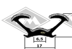
S35 (Glas/Rücken) Samtschiene befloct EUR 7,40/m*
