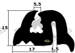
2069 Frontscheibenprofil EUR 5,70/m*
