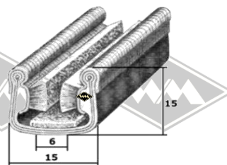
S119 Samtschiene mit Metalleinlage EUR 7,90/m*
